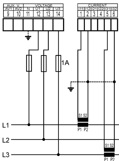
Síť IT Přímé Aronovo připojení ("3A")
