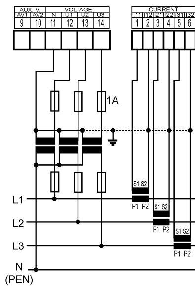
Síť TN Připojení do hvězdy ("3Y") přes PTN
