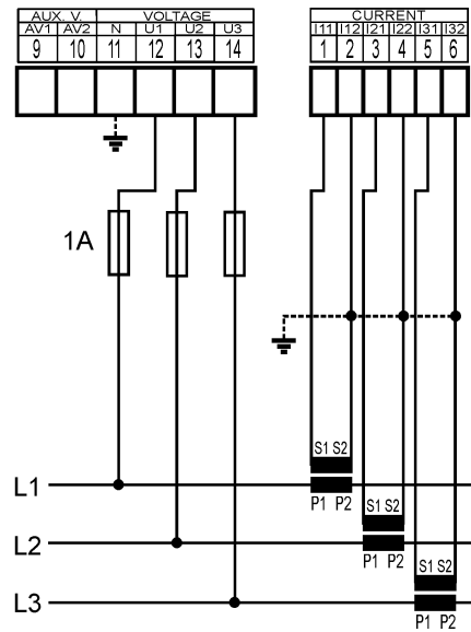
Síť IT Přímé připojení do trojúhelníka ("3D")
