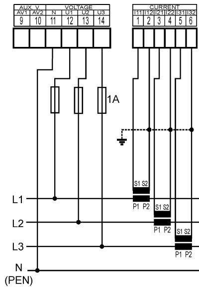
Síť TN Přímé připojení do hvězdy ("3Y")
