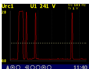
Obr. 4.11 : Graf signálu HDO
