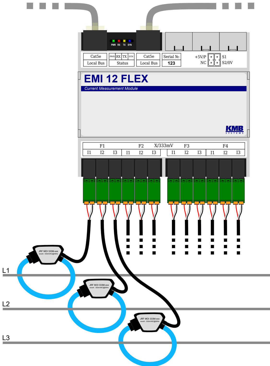
Obrázek 4: Příklad připojení proudových snímačů k modulu EMI 12.
