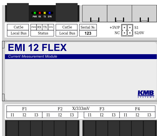
Obrázek 1: EMI 12 S FLEX
